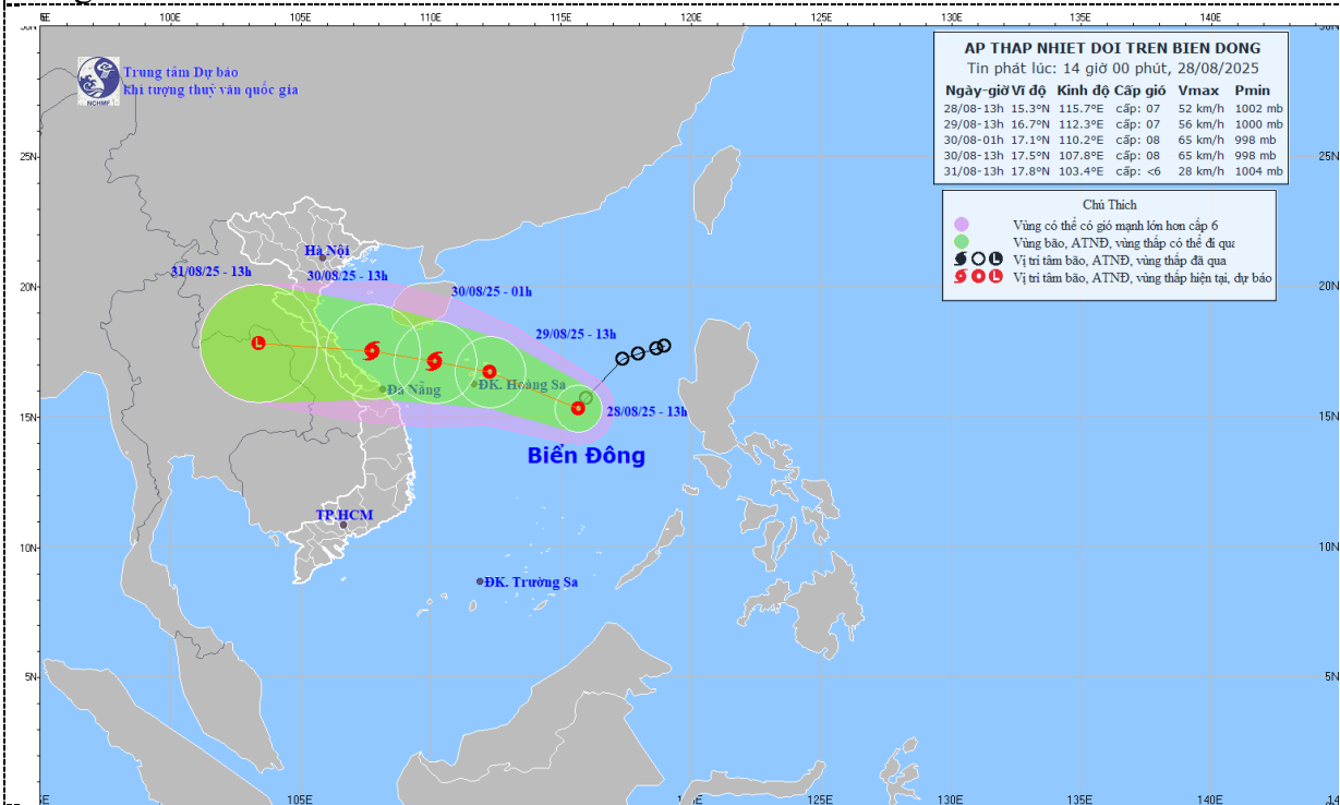
Hình1. Bản đồ dự báo quỹ đạo và cường độ áp thấp nhiệt đới phát lúc 14h00 ngày 28/8/2025
