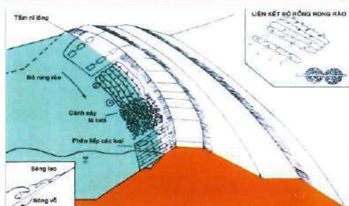
Giảm bớt chiều cao sóng leo - Hạn chế sức phá của sóng
