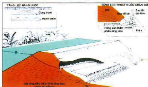
Cử chân chống sụt - Thoát nước, đắp cơ
