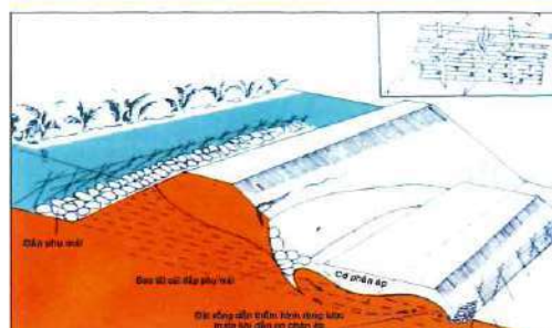
Áp trước mái trước - Đắp cơ chống trượt - Rút nước mái sau
