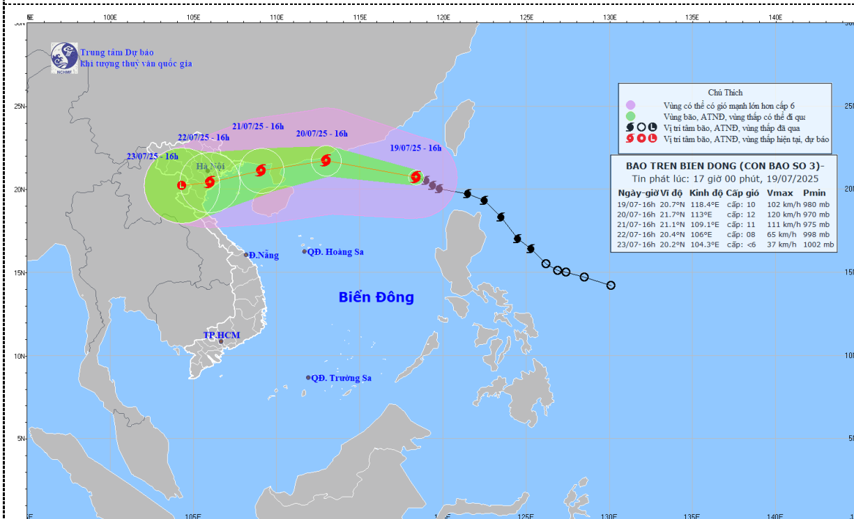
Hình1. Bản đồ dự báo quỹ đạo và cường độ bão số 3 phát lúc 17h00 ngày 19/7/2025
