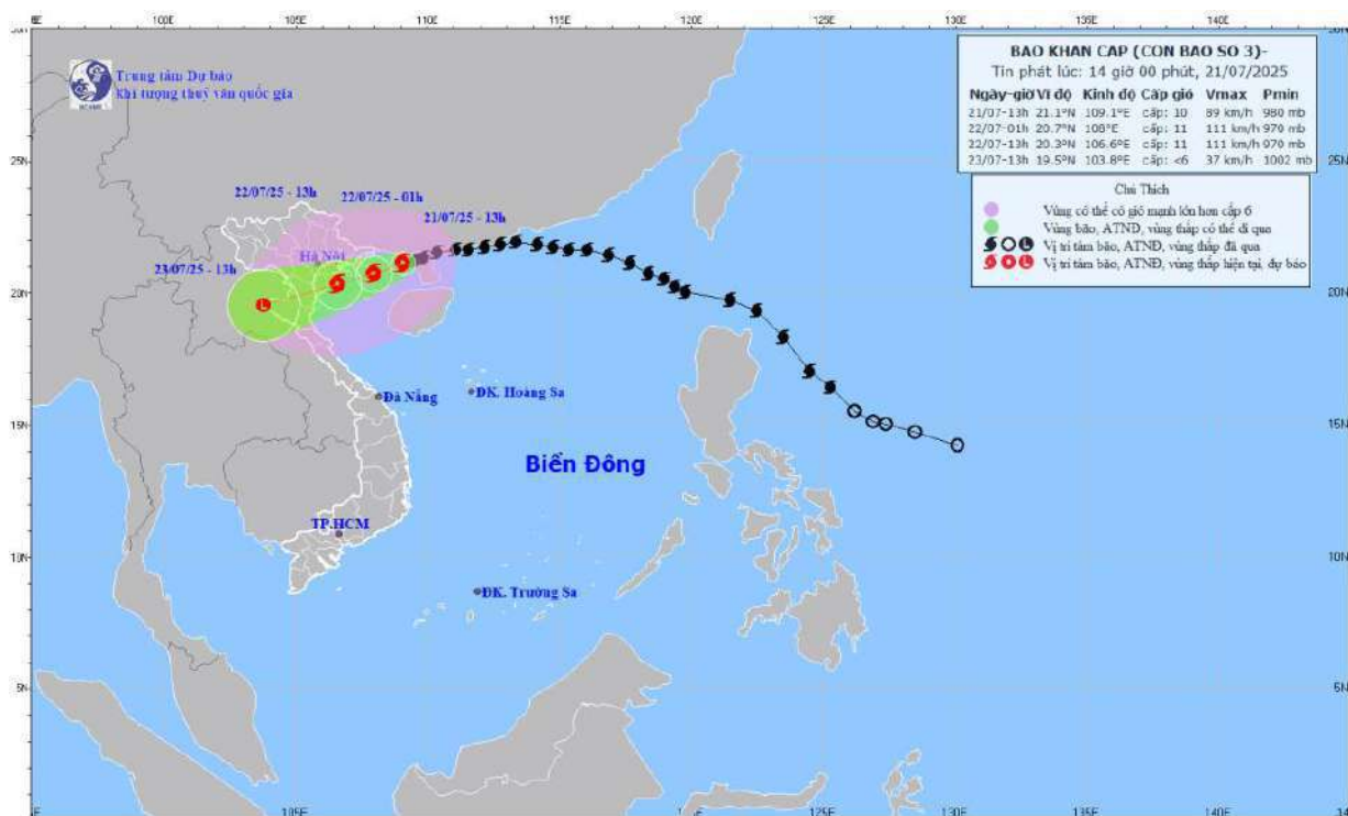
Hình1. Bản đồ dự báo quỹ đạo và cường độ bão số 3 phát lúc 1400 ngày 21/7/2025
