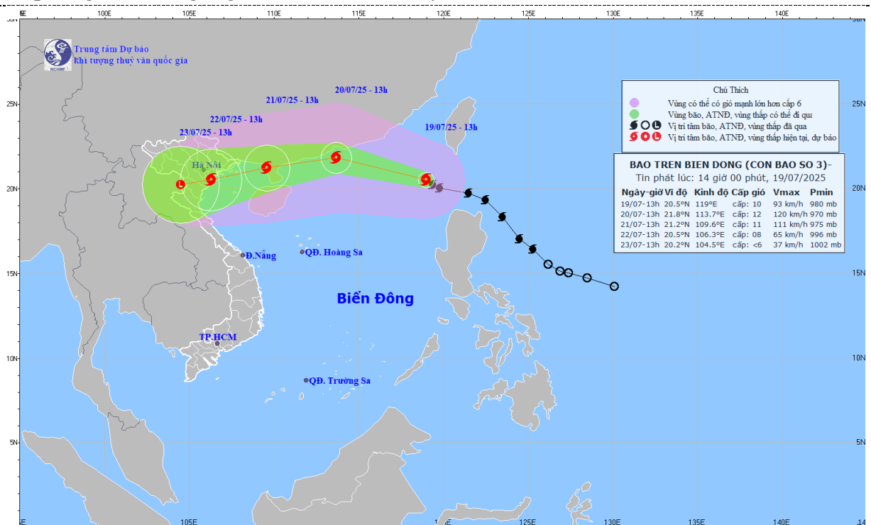
Hình 1. Bản đồ dự báo quỹ đạo và cường độ bão Wipha phát lúc 14h00 ngày 19/7/2025
