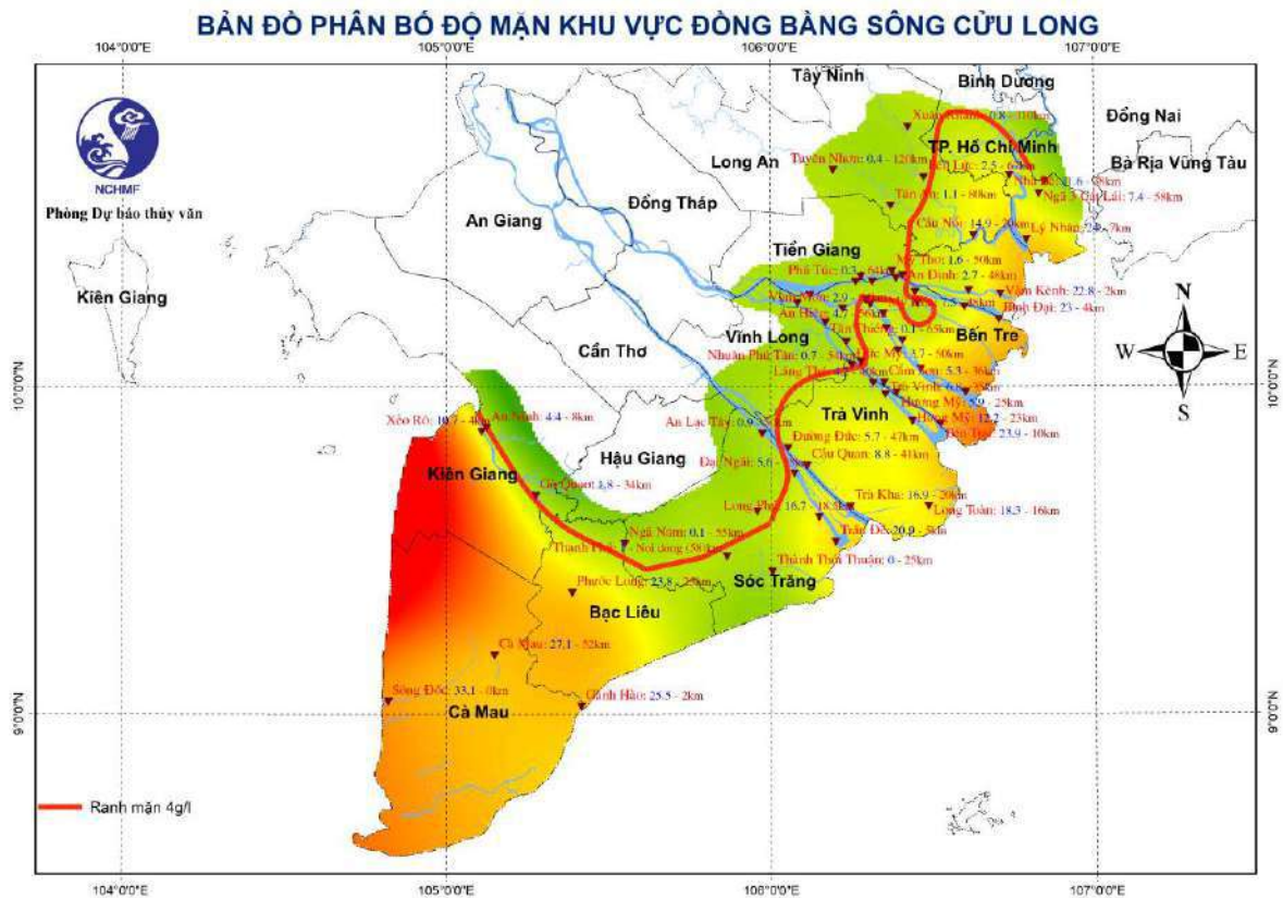
Hình 3. Bản đồ phân bố độ mặn từ 11-20/3/2025
