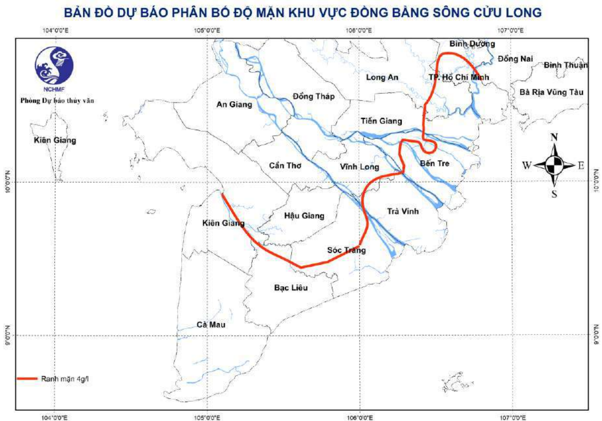
Hình 4. Bản đồ dự báo phân bố độ mặn cao nhất từ 21-31/3/2025
