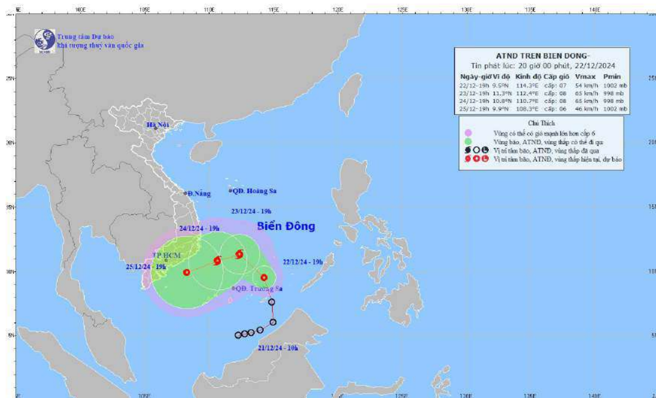
Bản đồ dự báo quỹ đạo và cường độ ATNĐ phát lúc 20h00 ngày 22/12/2024
