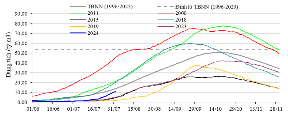
Hình 6. Diễn biến dung tích Biển Hồ đến ngày 01/8/2024
