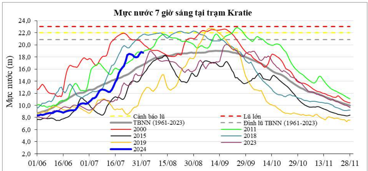
Hình 4. Diễn biến mực nước tại Kratie đến ngày 01/8/2024
