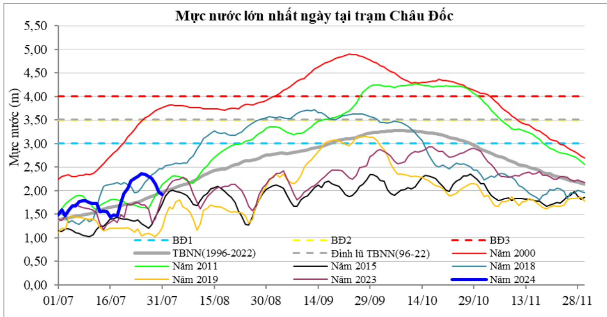
Hình 8. Diễn biến mực nước tại trạm Châu Đốc đến ngày 31/7/2024
