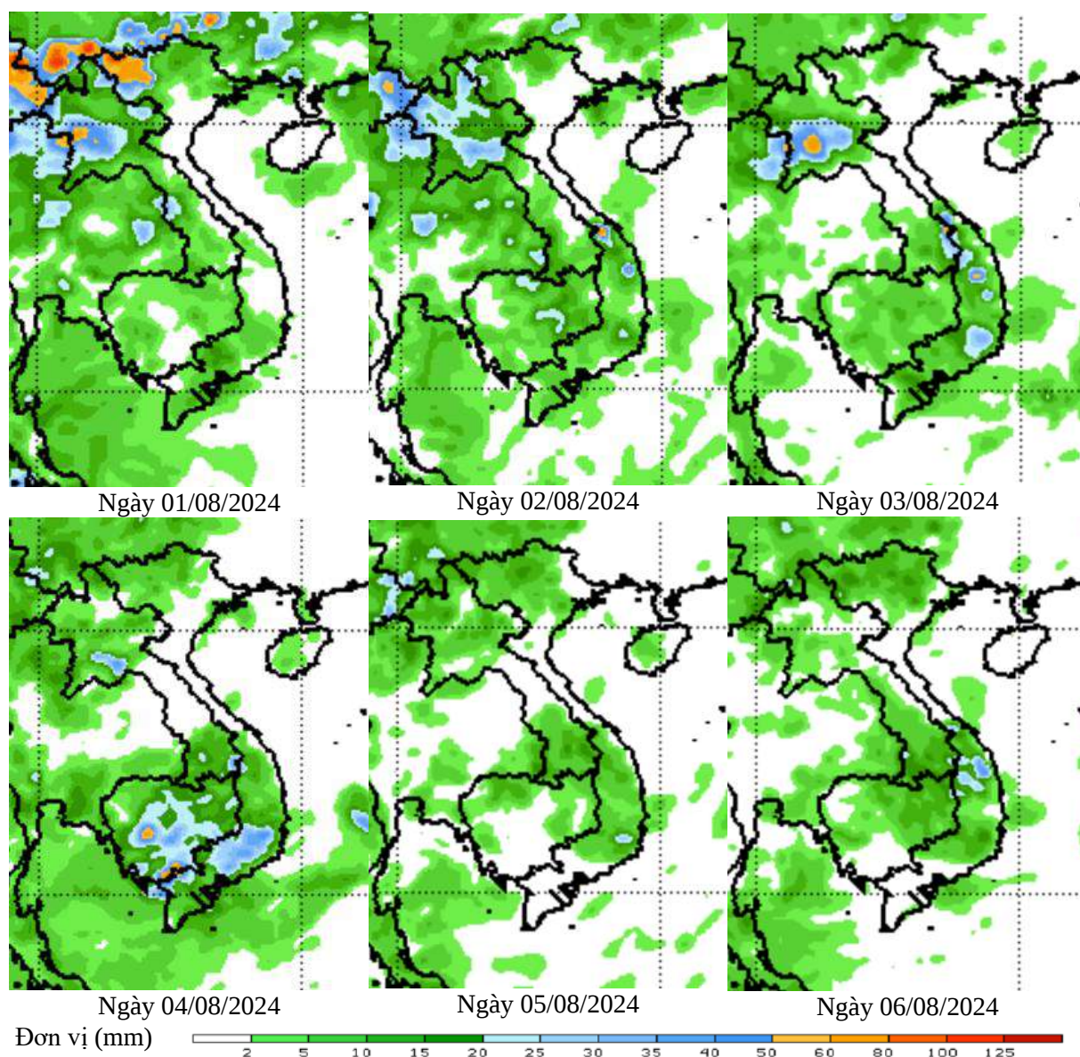
Hình 10. Dự báo mưa từ ngày 01/8 - 06/8/2024 khu vực hạ lưu sông Mê Công
