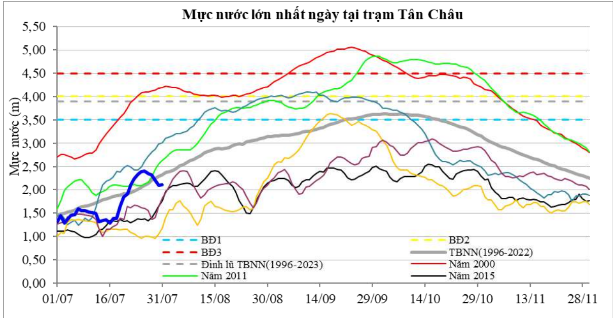
Hình 7. Diễn biến mực nước tại trạm Tân Châu đến ngày 31/7/2024
