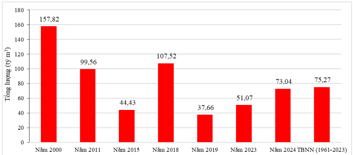
Hình 3. Tổng lượng lũ tại Kratie từ 01/6 đến ngày 25/7/2024
