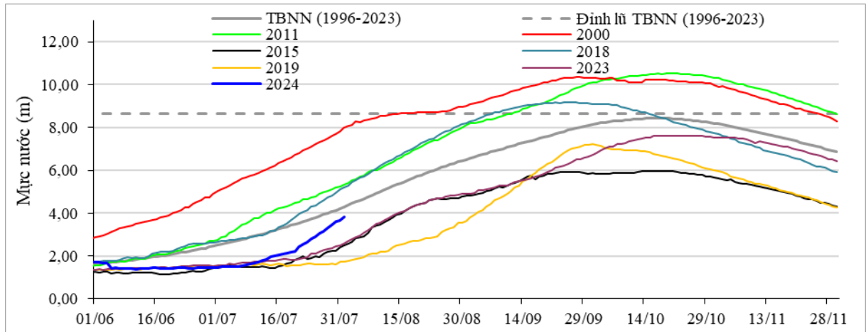
Hình 5. Diễn biến mực nước Biển Hồ đến ngày 01/8/2024
