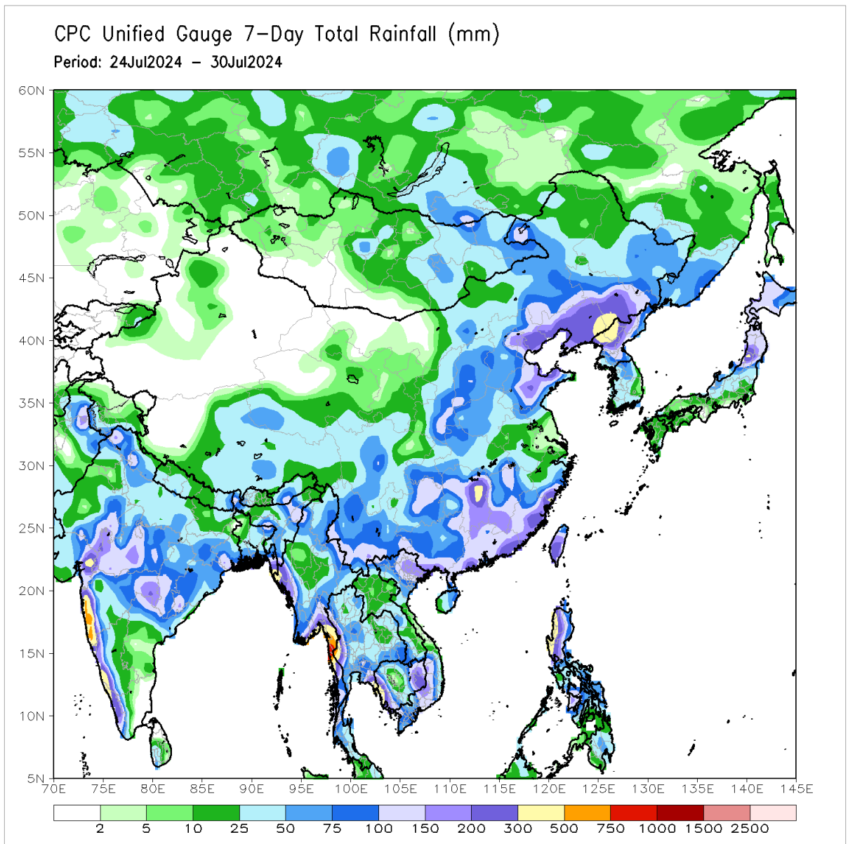
Hình 2. Bản đồ mưa lũy tích tuần từ 24/7 - 30/7/2024 trên lưu vực sông Mê Công
