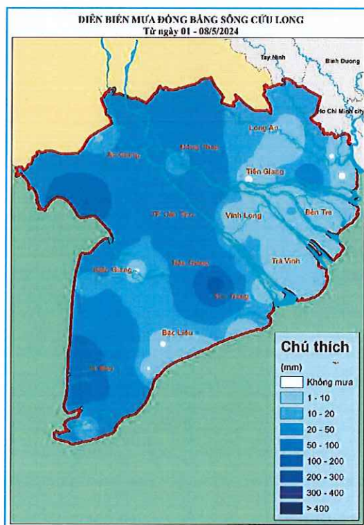
Hình 4. Bản đồ lũy tích lượng mưa trên vùng DBSCL (từ ngày 01 đến 08/5/2024)
