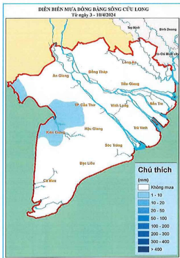
Hình 4. Bản đồ lũy tích lượng mưa trên vùng ĐBSCL (từ ngày 03/04 đến 10/4/2024)
