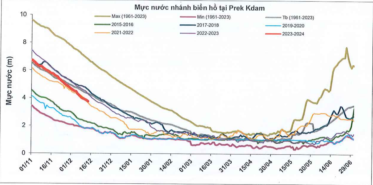
Hình 1. Diễn biến mực nước trạm Prek Kdam - Biển hồ, cập nhật ngày 13/12/2023
