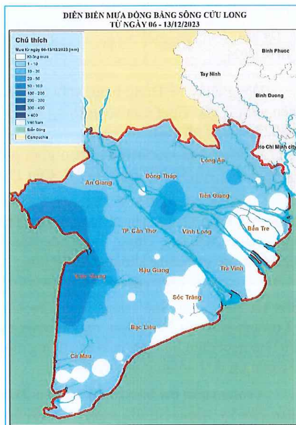
Hình 4. Bản đồ lũy tích lượng mưa trên vùng ĐBSCL (từ ngày 06/12 đến 13/12/2023)
