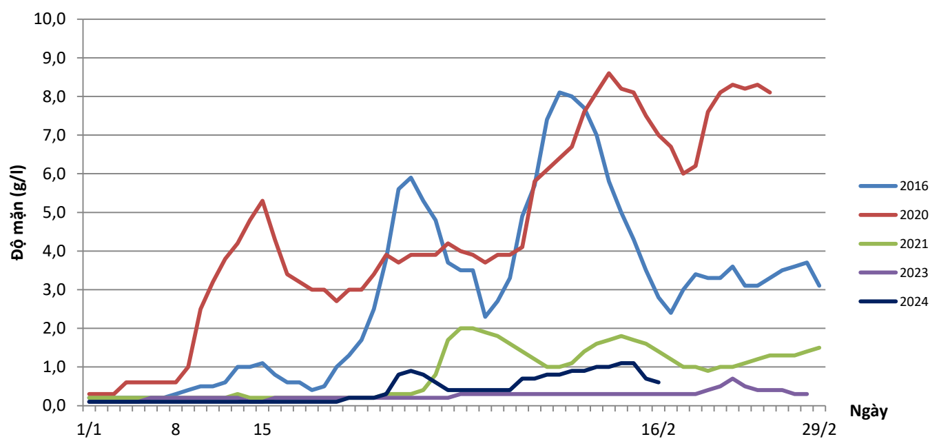
Biểu đồ độ mặn sông trạm Tân An (sông Vàm Cỏ)
