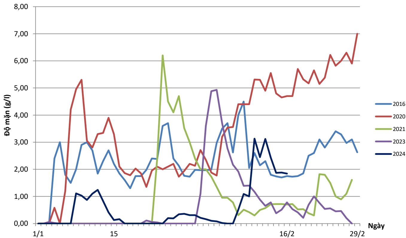
Biểu đồ độ mặn sông trạm Xuân Hòa (sông Tiền)
