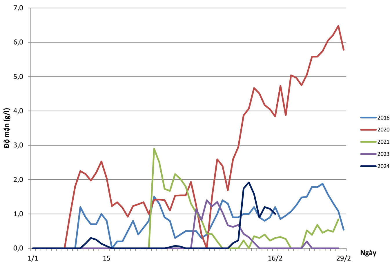
Biểu đồ độ mặn sông trạm Vườn hoa Lạc Hồng (sông Tiền)
