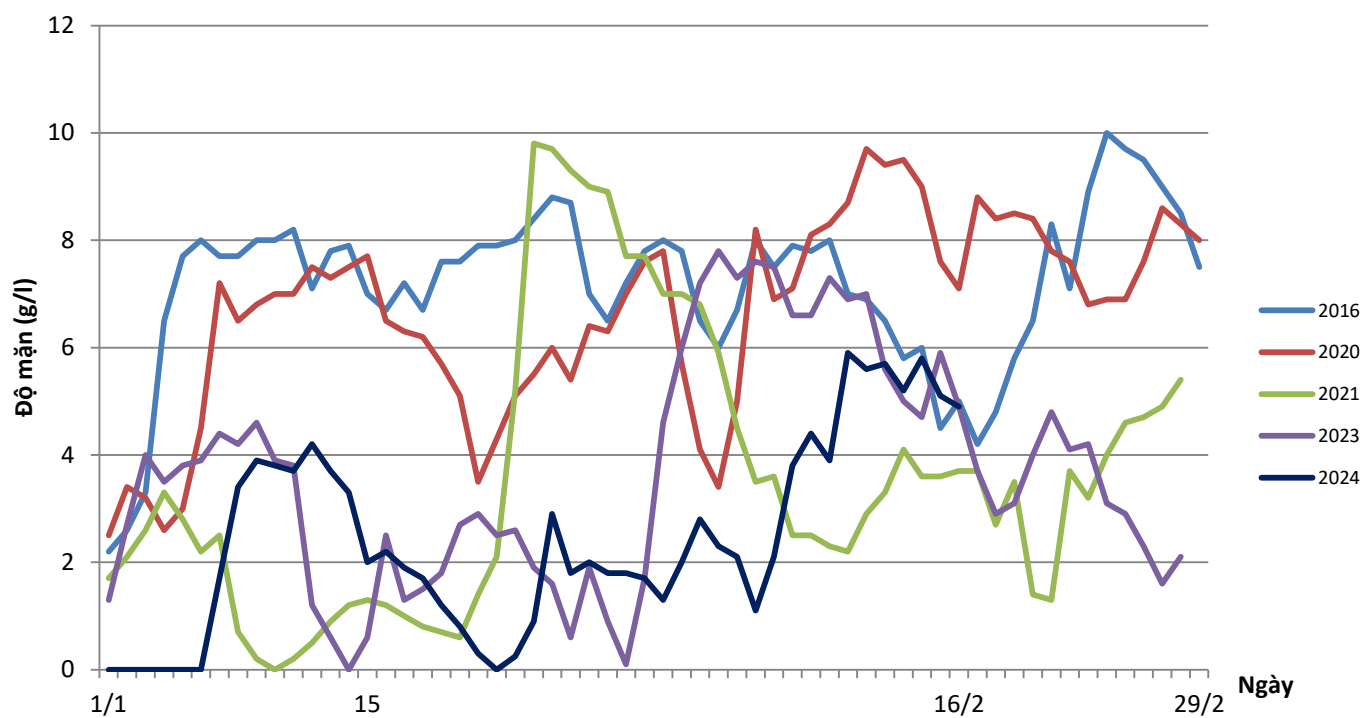
Biểu đồ độ mặn sông trạm Vàm Giồng (sông Tiền)
