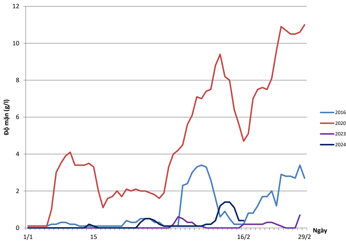
Biểu đồ độ mặn sông trạm Vàm Môn (sông Hàm Luông)
