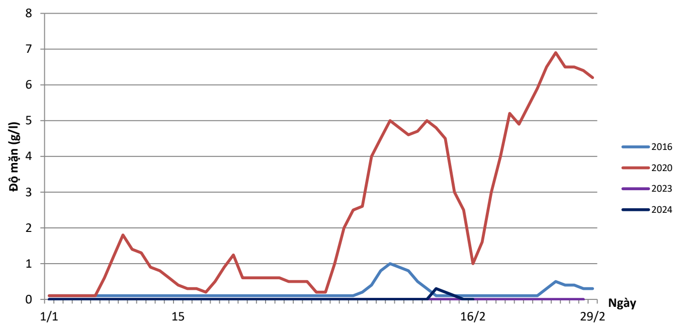
Biểu đồ độ mặn sông trạm Hòa Nghĩa (sông Hàm Luông)
